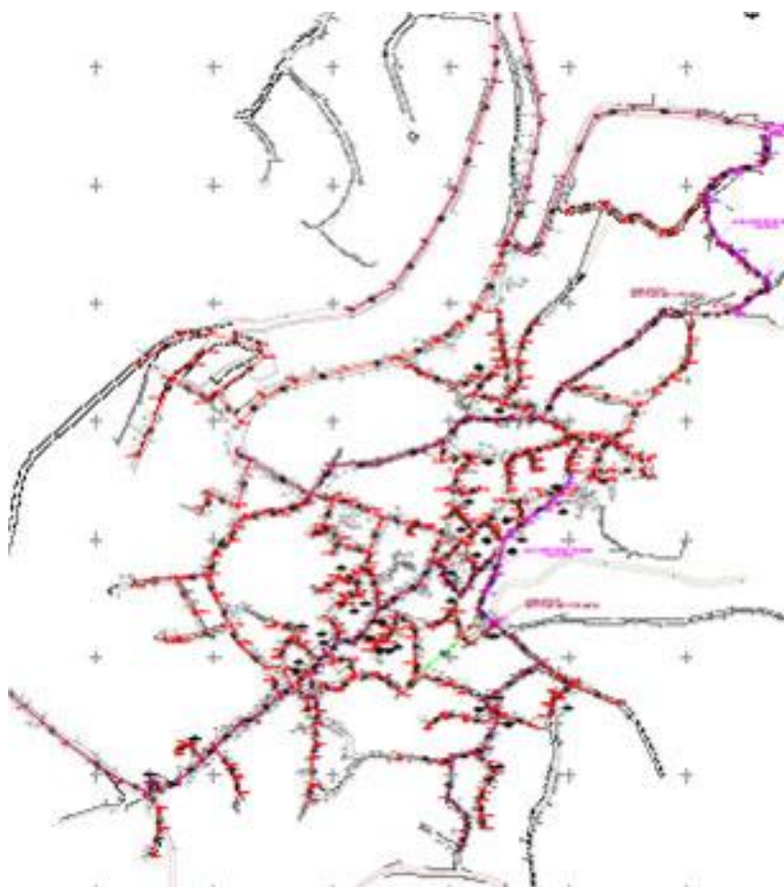
Κάτοψη δικτύου αποχέτευσης Οικισμού Λευκών
